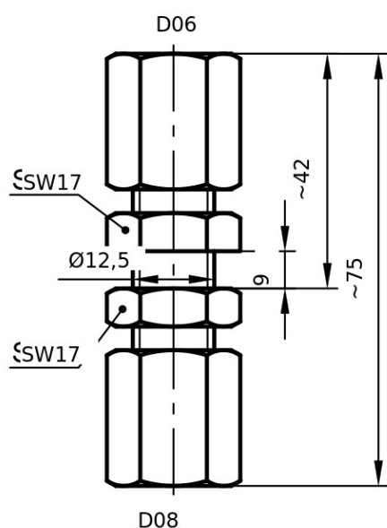
Valori espressi in mm; Illustrazione esemplare
