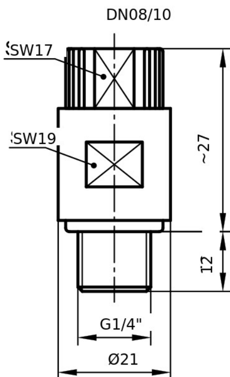
Valori espressi in mm; Illustrazione esemplare
