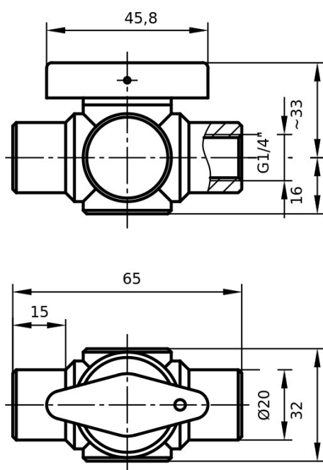
單位測量以毫米 (mm) ; 示例說明
